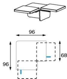
FL 009 hoekelement met blad
