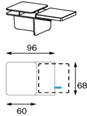
FL 006 eindelement met dubbeldeks blad
