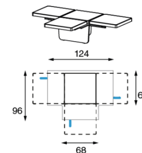
FL 012 t-element inclusief 1 zitkussen
