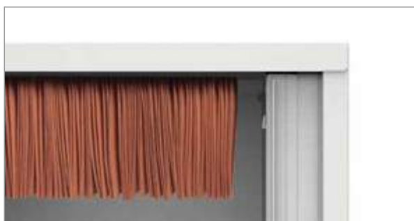
Rail bovenaan in de kast voor lateraal klassemment Rail dans la tête pour classement latéral.
